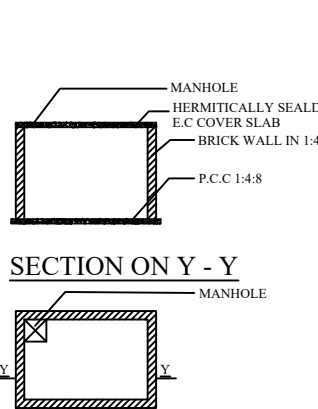
UG - SUMP DATAIL PLAN
