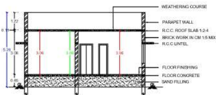
SECTION A-B
