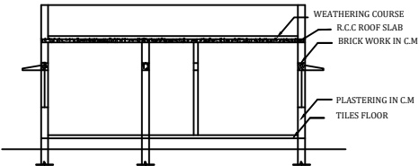
SECTION 'ab'
