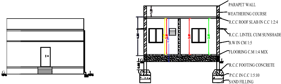
ELEVATION
