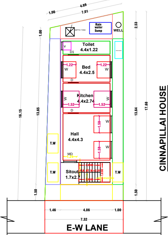
SITE PLAN CUM
