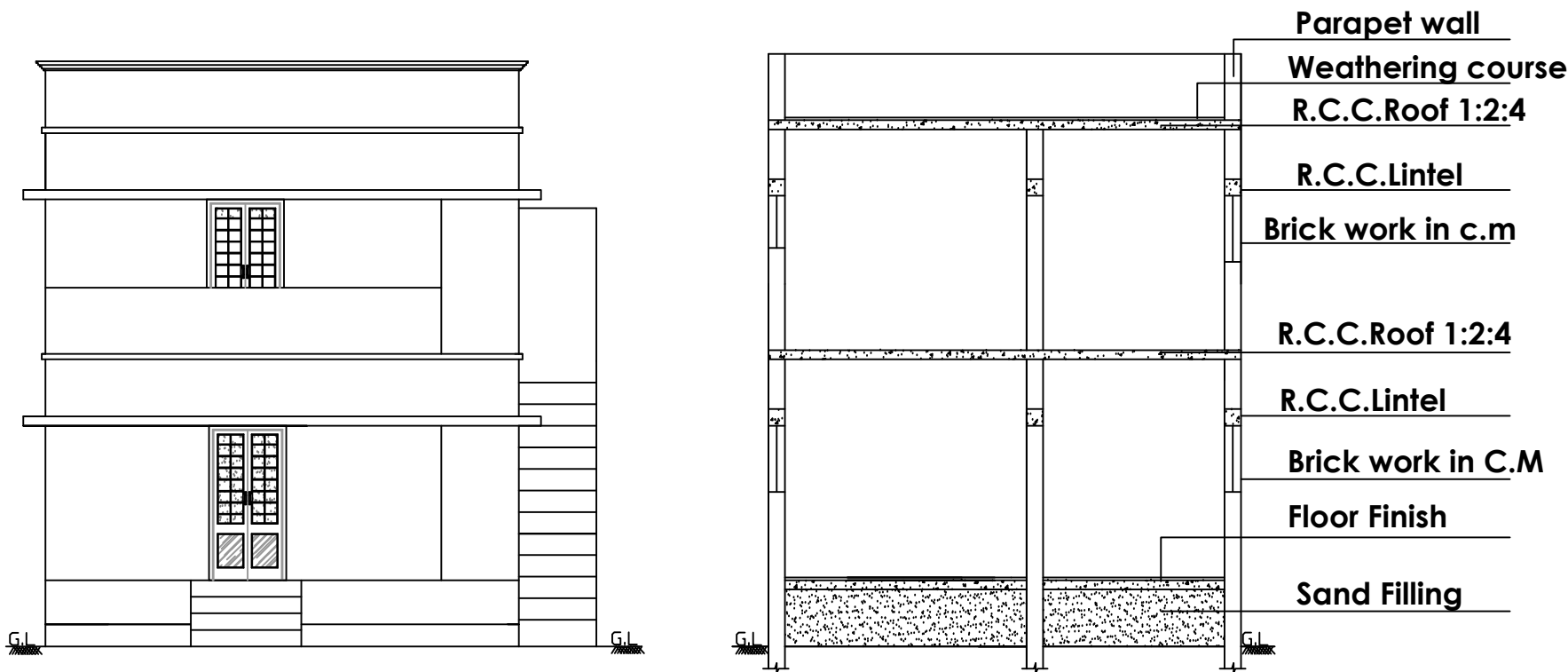
ELEVATION
