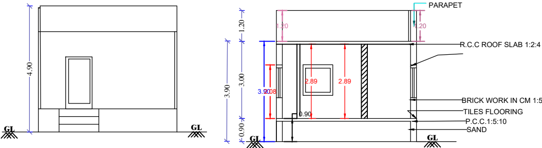
ELEVATION
