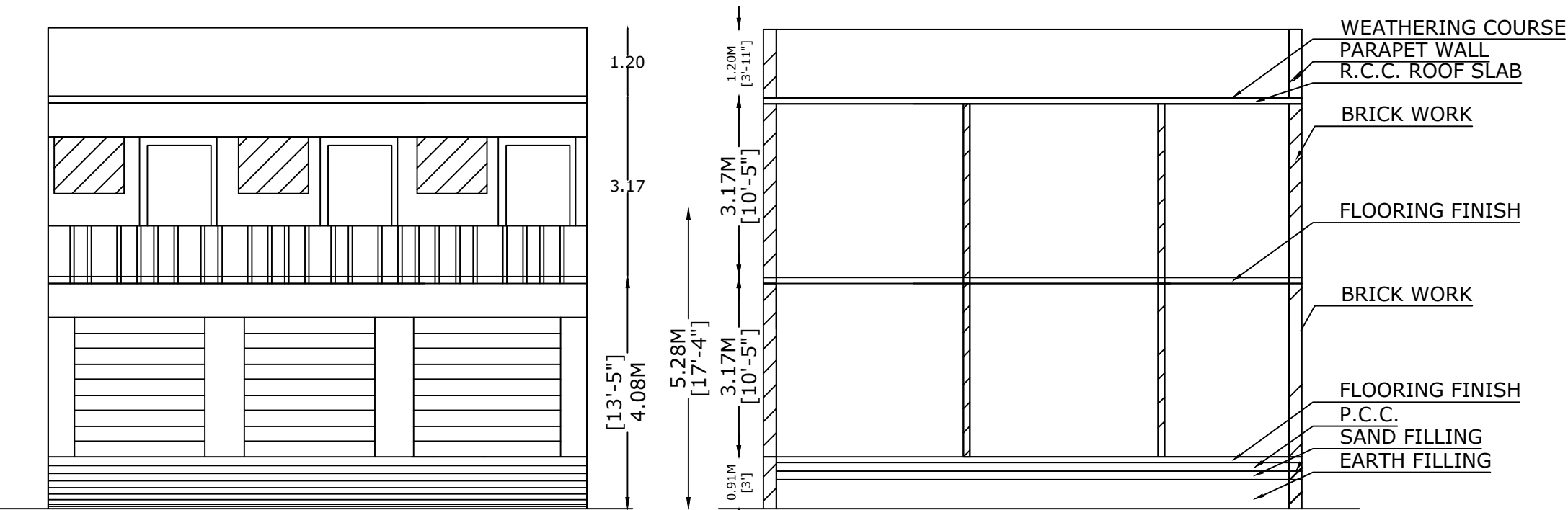
ELEVATION
