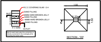
SECTION - C-D
