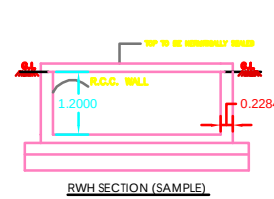
RW_CAPACITY_L=2000LTRS
