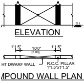
ELEVATION
