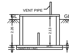
SECTION DD
