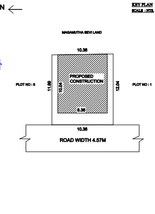
KEY PLAN SCALE : 1:250
