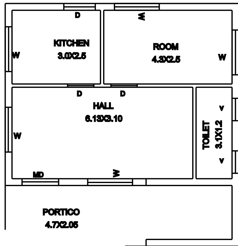
DOOR PLAN
