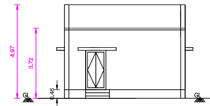
ELEVATION
