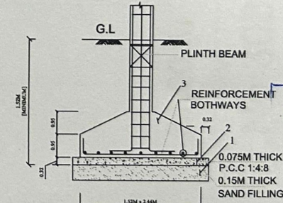
TYP. DET. COLUMN FOOTING
