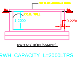
RWI SECTION (SAMPLE) RWI_CAPACITY_L=2000LTRS
