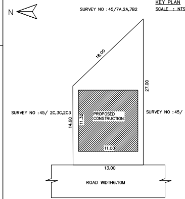
KEY PLAN SCALE : 1:500
