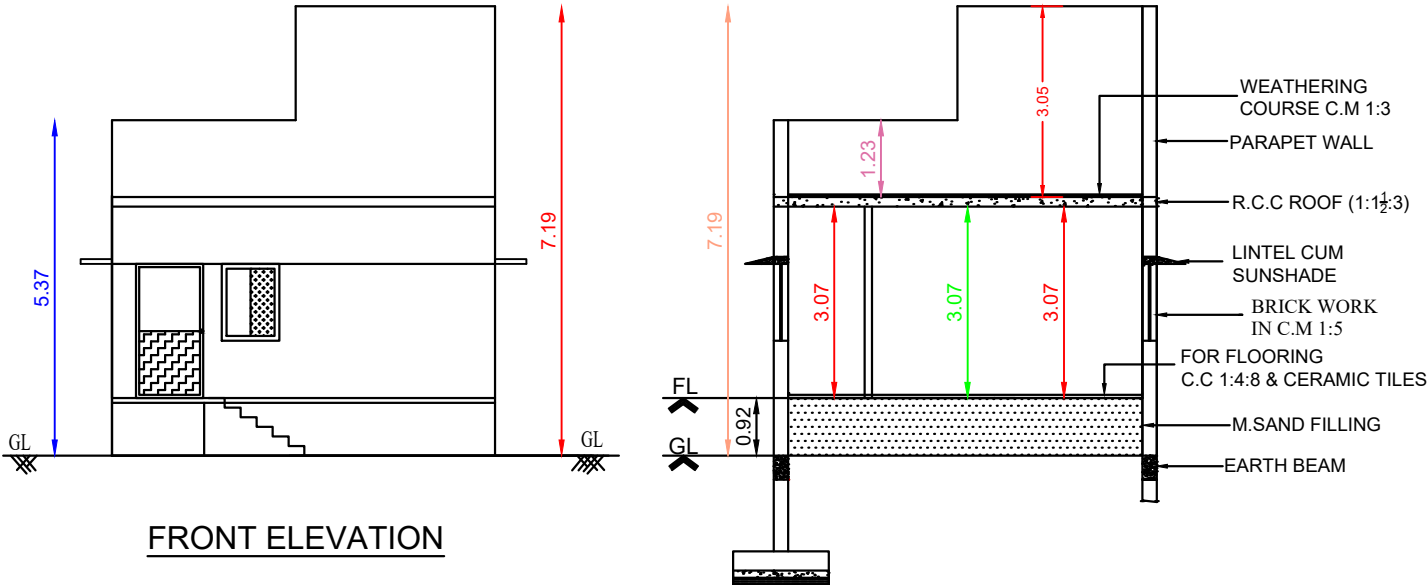
SECTION ON(A-A)
