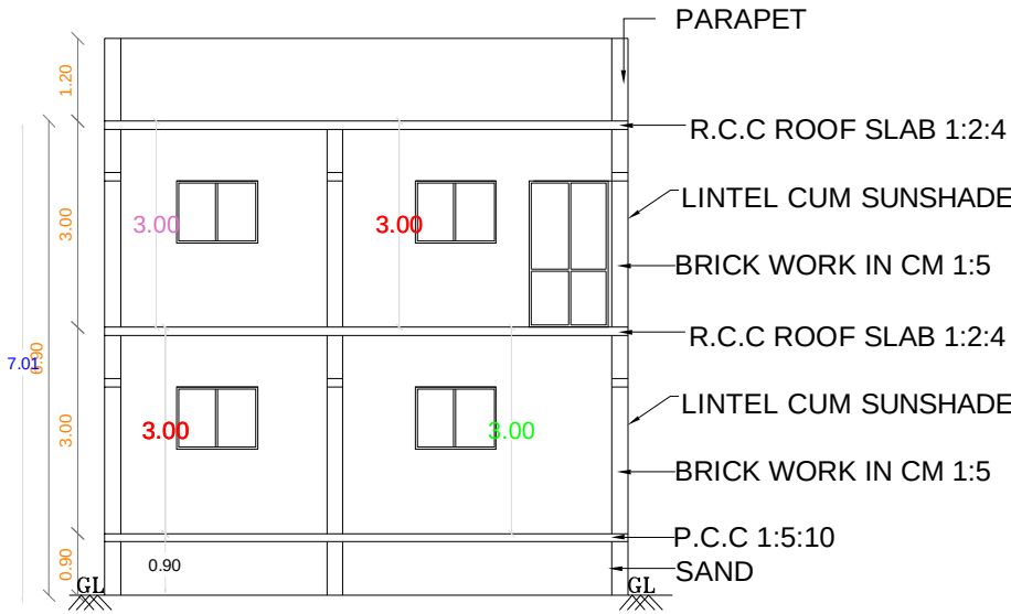
SECTION A-A
