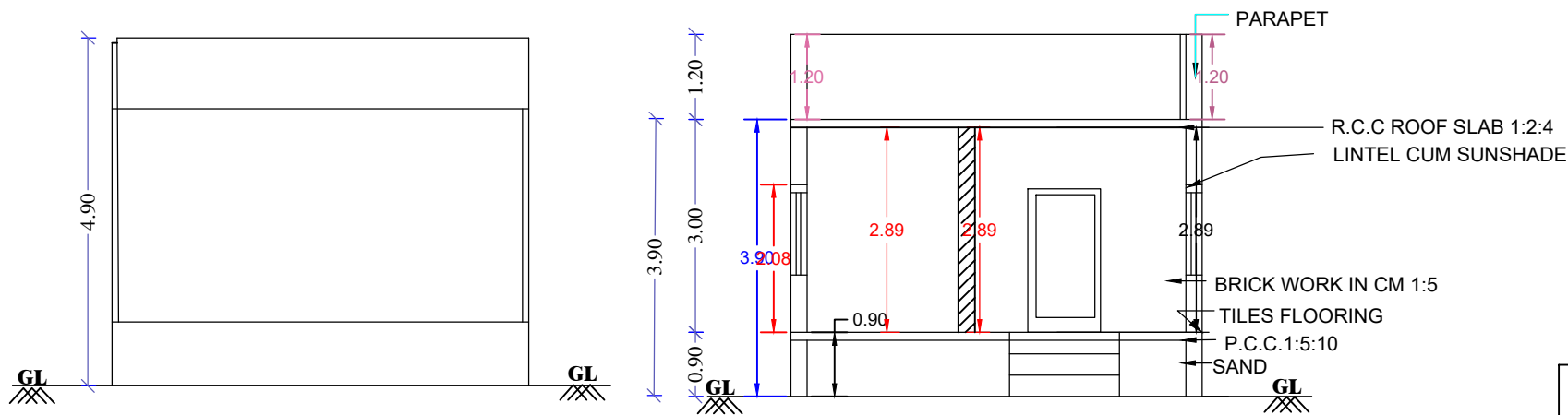
ELEVATION
