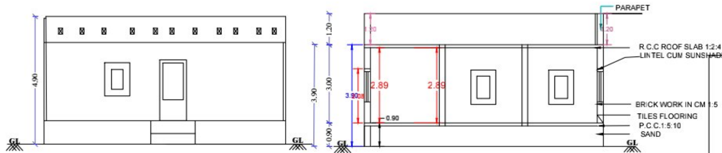
ELEVATION
