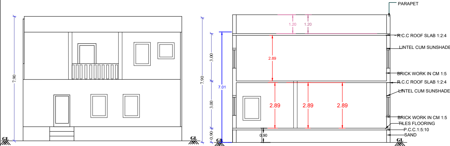
ELEVATION
