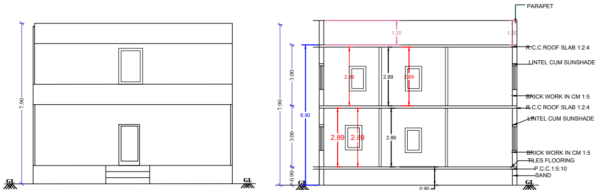
ELEVATION
