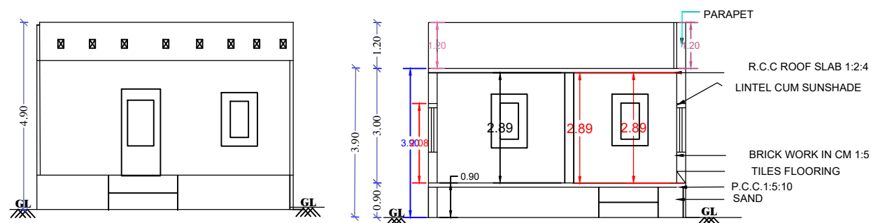
ELEVATION
