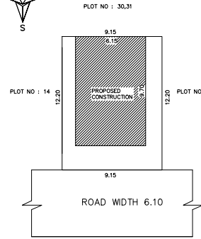
KEY PLAN SCALE : 1:100
