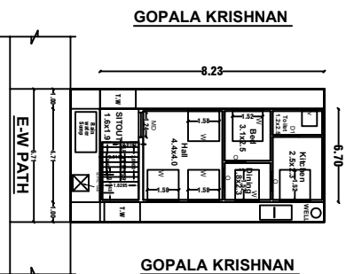
SITE PLAN CUM
