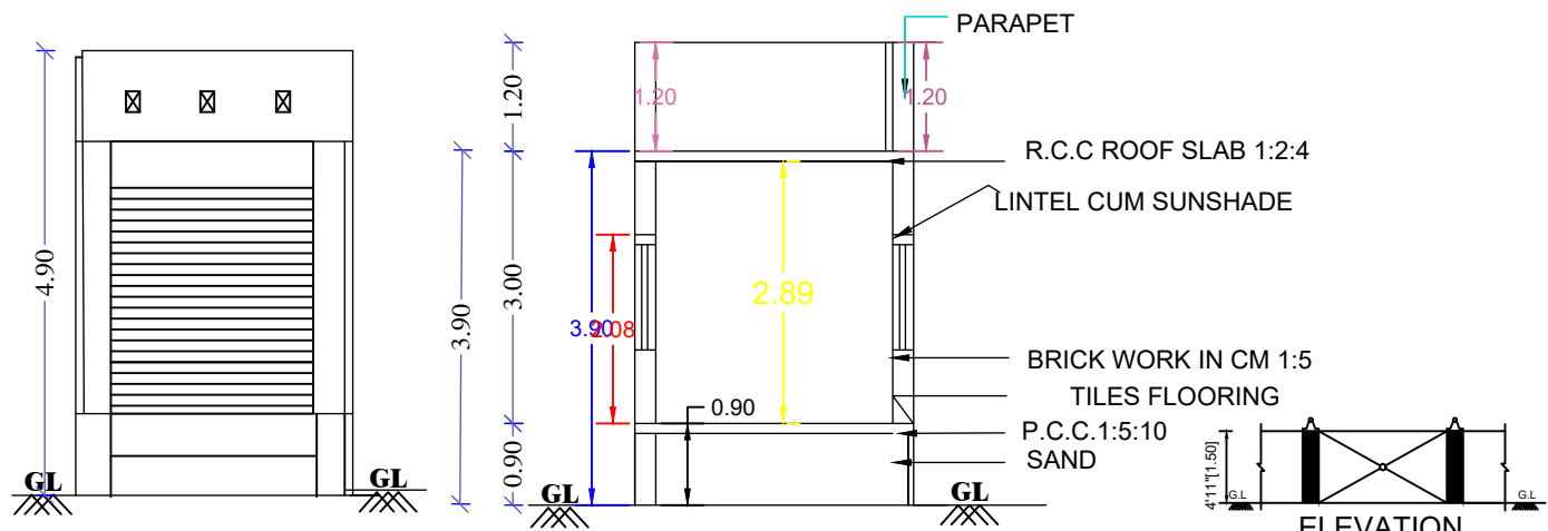
ELEVATION
