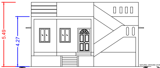
ELEVATION
