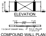
ELEVATION
