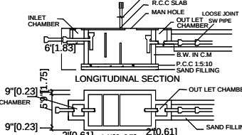
LONGITUDINAL SECTION
