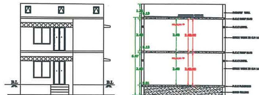
ELEVATION
