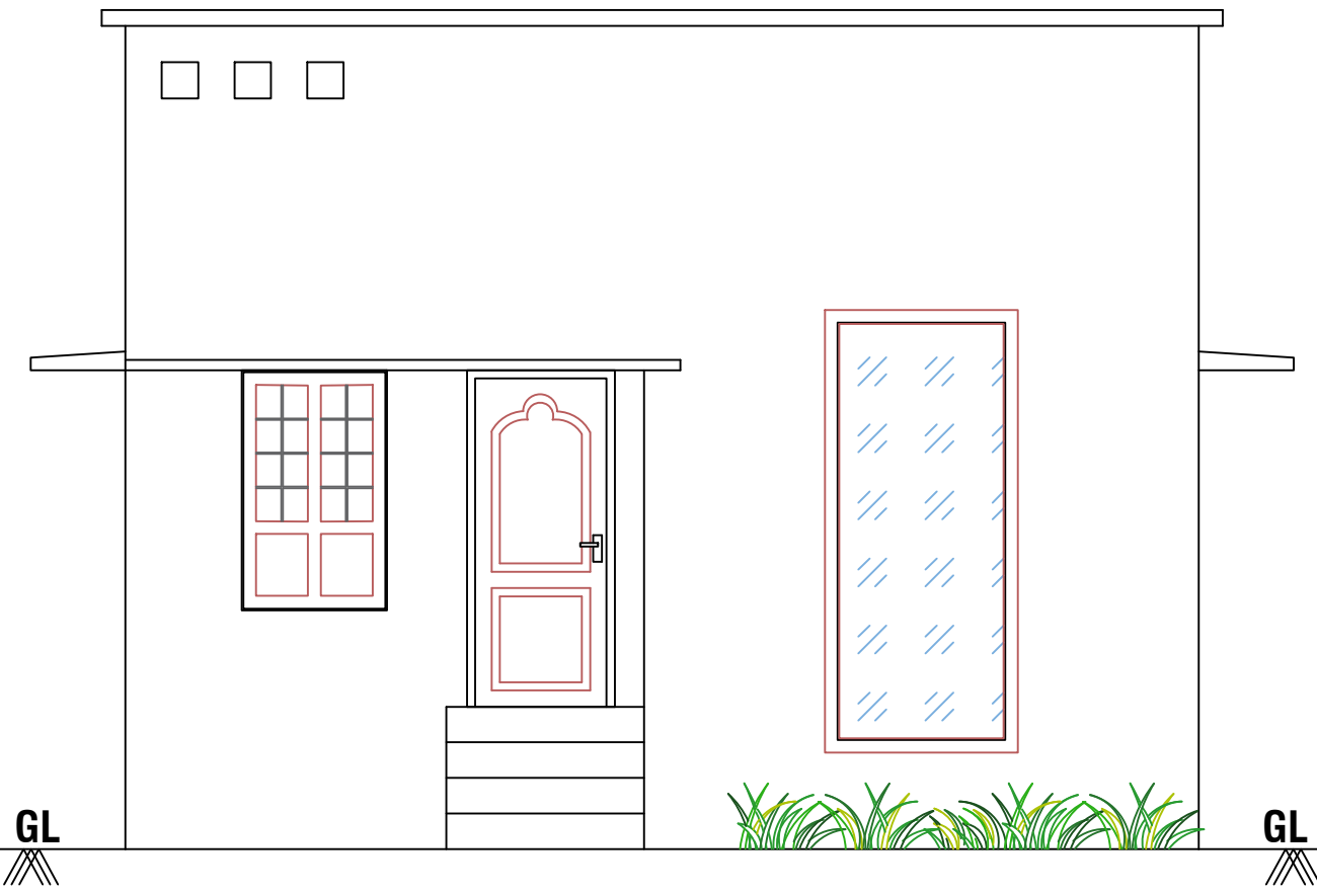
ELEVATION
