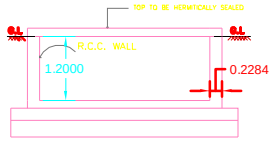
RWK SECTION (SAMPLE)
