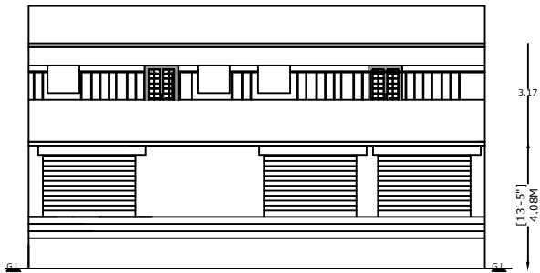
ELEVATION
