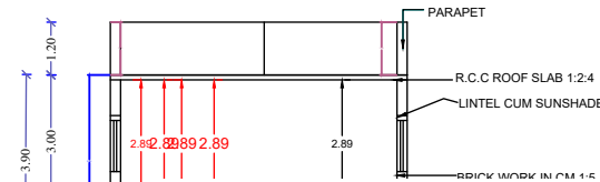
ELEVATION
