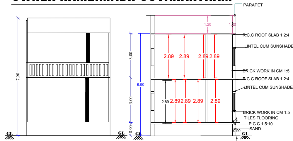
ELEVATION
