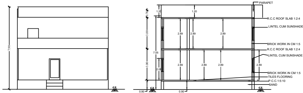
ELEVATION
