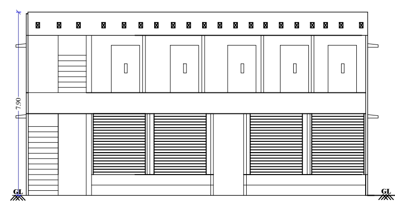
ELEVATION
