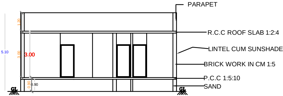
SECTION A-A
