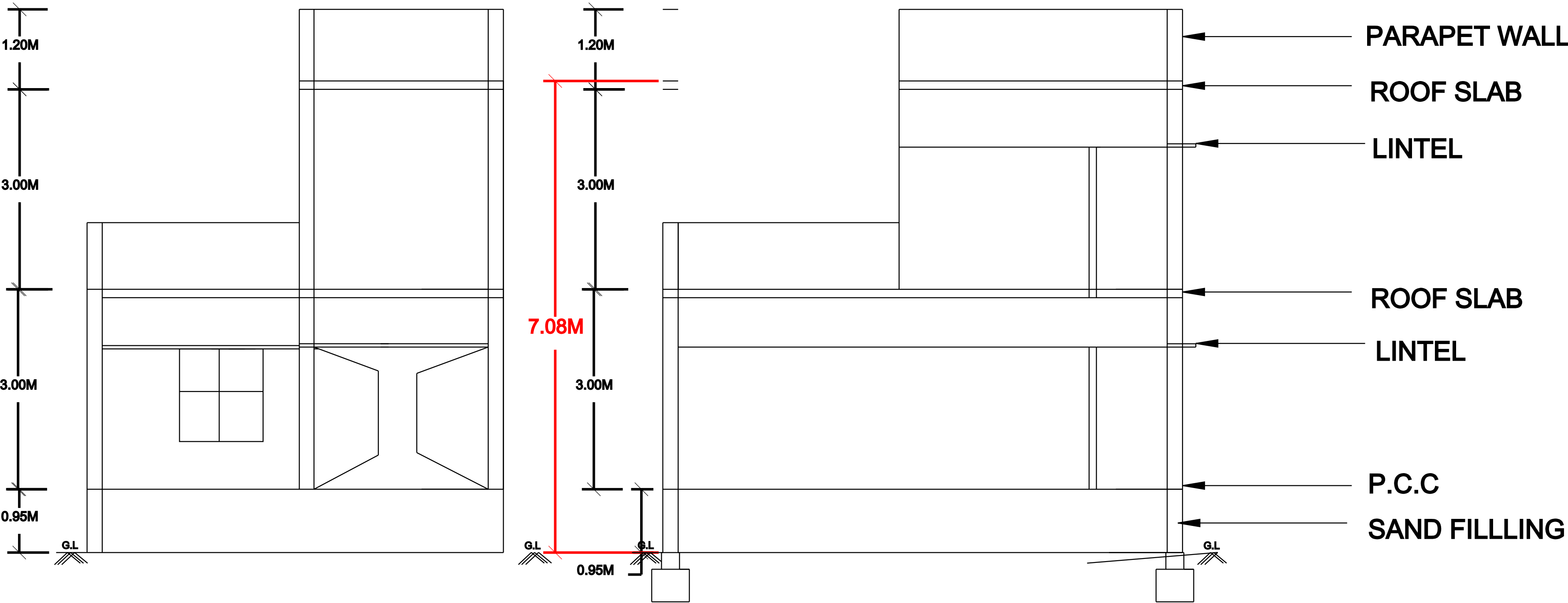
ELEVATION
