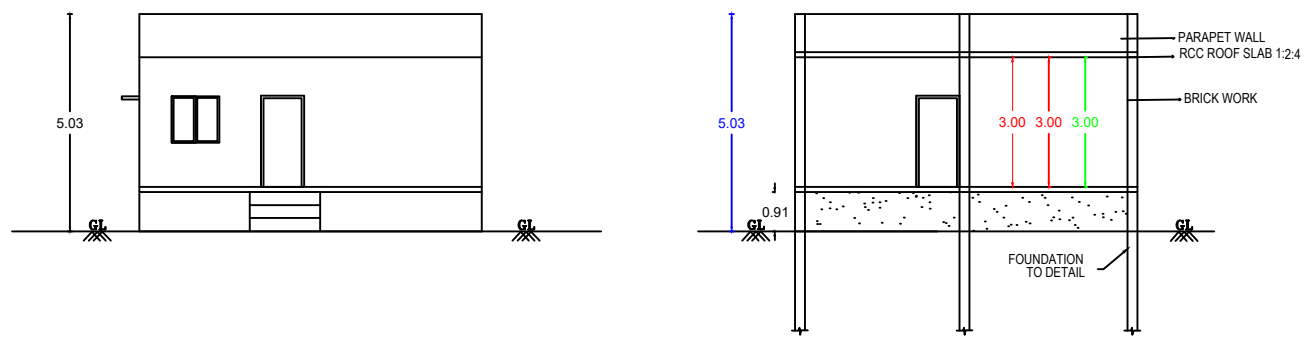
ELEVATION
