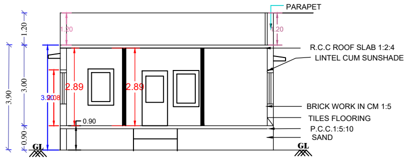
SECTION A-B
