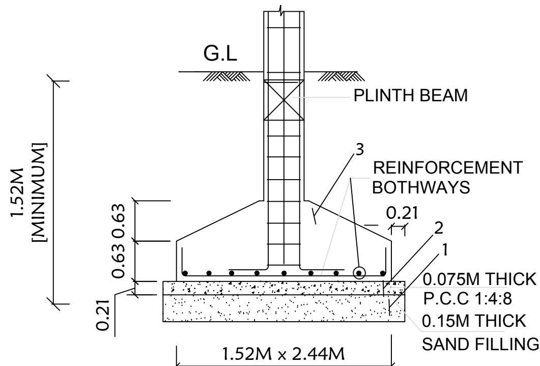
TYP. DET. COLUMN FOOTING
