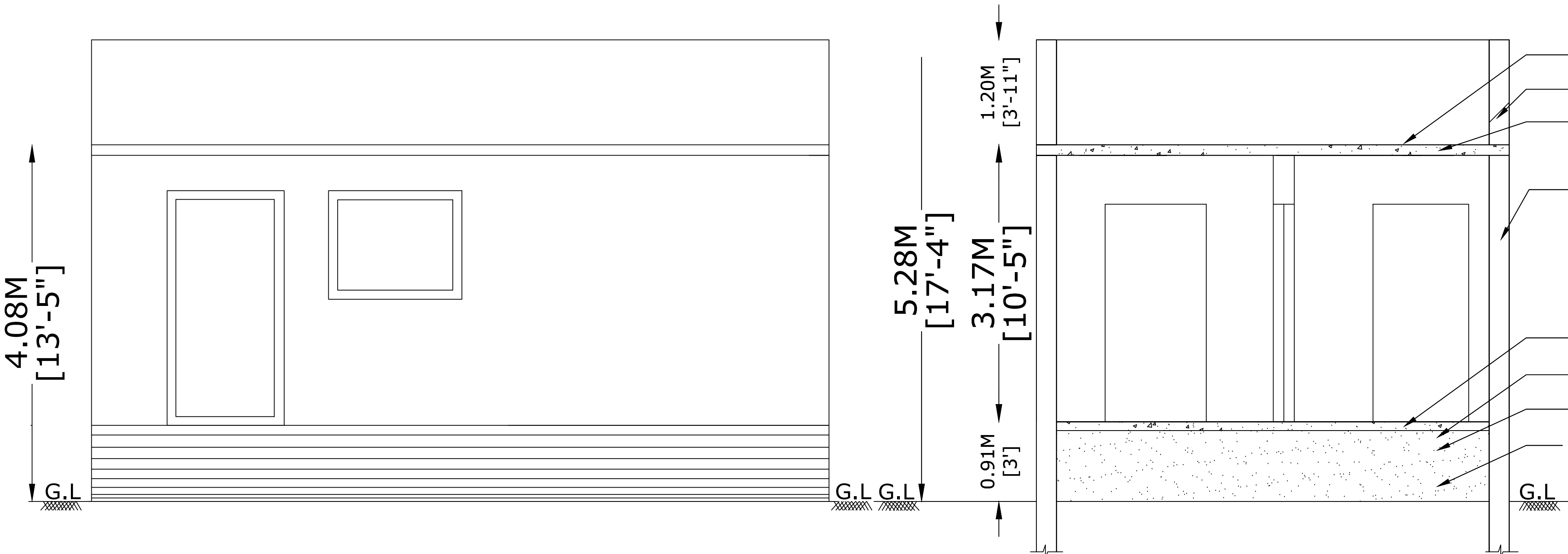
ELEVATION
