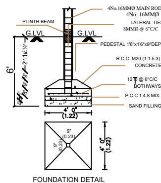
FOUNDATION DET.
