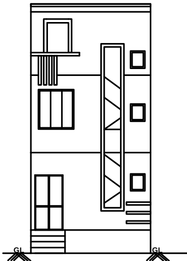
ELEVATION
