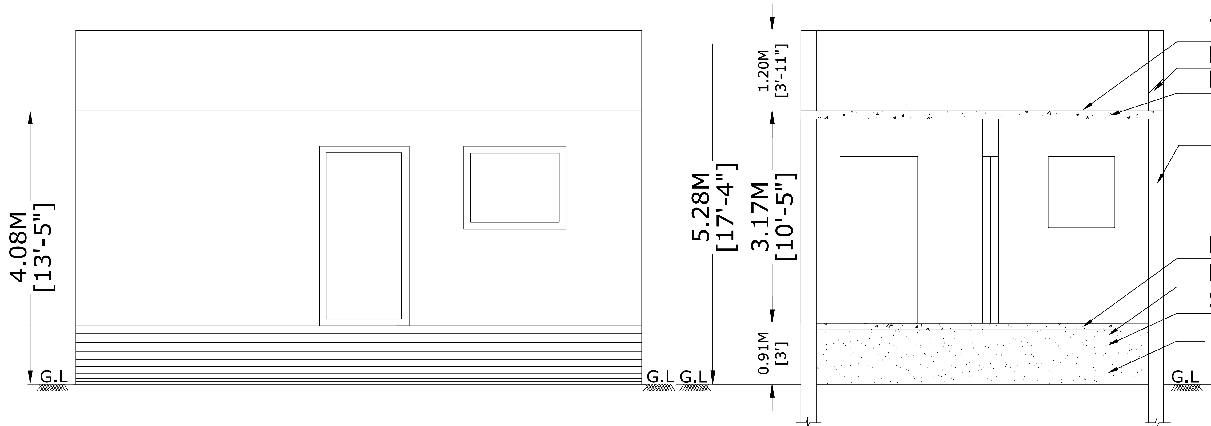
ELEVATION
