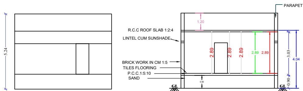
ELEVATION
