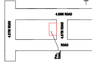
SITE PLAN SCALE-1:100
